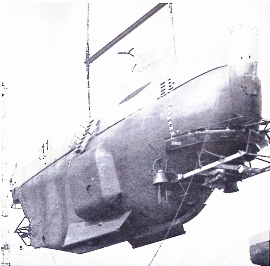
Den vældige flyder med benzin. I bagenden ses skruen til fremaddrift, i forenden en halvcirkel med projektorene og derunder den vandrette ramme, hvorpå samlegrabben kører. Passagerkuglen sidder, hvor kolen bøjer opetter
