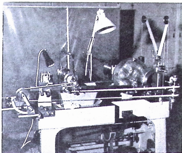
Formindskelsesmaskinen. Til højre den store oprindelige broncemodel
