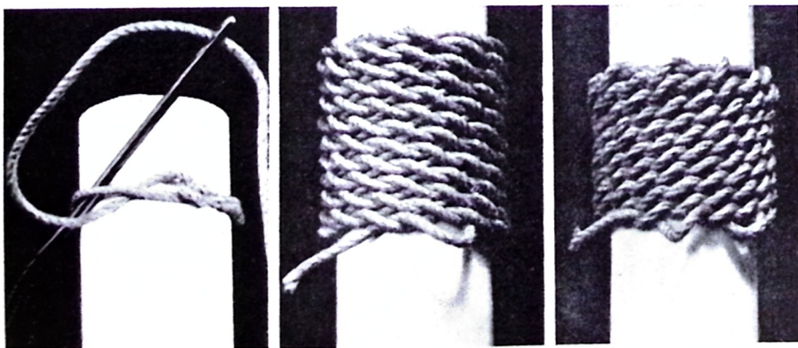
Fig. 2. Til venstre ser man påbegyndelse af katning med et splejset øje på garnets ene ende. Med garnet er taget en rundtørn helt omkring den genstand, der skal klædes, og garnets anden tamp er trukket gennem øjet. Ved hjælp af nålen lægges nu rundtørner omkring det første garn. Billedet i midten viser fortsættelse af overhånds rundtørner gennem bugterne i den foregående række rundtørner. Til højre vises garnets føring i underhånds rundtørnskatning.
