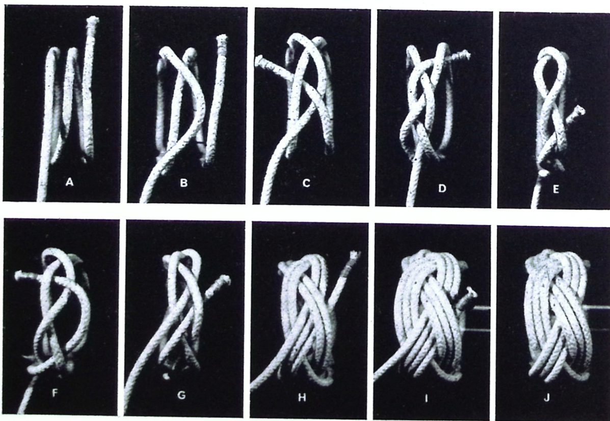
Fig. 2. Således fremstilles det ringformede, treslåede tyrkerknob med fem bugter.
