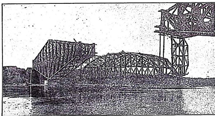
Quebec-Broen over St. Lawrencefloden i Kanada med Verdens største Brospænd under Opførelse.
