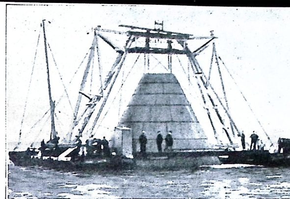
Tragten er anbragt over det Sted, hvor Vraget ligger, para til at blive sænket. Der kan arbejdes inde i Tragten uden Dykkerhjelme.
