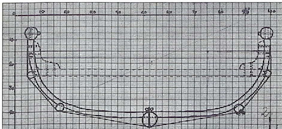
2. tværsnit og spanterids.
