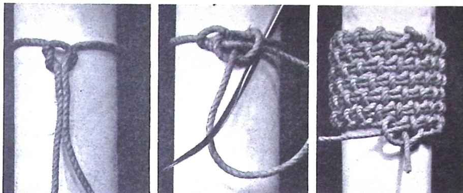
Fig. 4. Den almindelige fremgangsmåde ved åben halvstikskatning over medløber, hvor medløberen har samme tykkelse som arbejdsgarnet.
