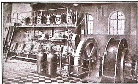
Elektricitetsværk med Jævnstrømsgenerator; fra venstre ses: Dieselmotor, Svinghjul og Dynamo.
