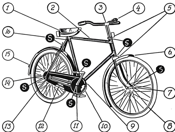
Cyklens Dele: 1. Sadel, 2. Stel, 3. Styr, 4. Klokke, 5. Styrelejer, 6. Skærme, 7. Forhjulsnæv, 8. Fælg, 9. Oliebadskædekasse, 10. Tandhjul, 11. Krank, 12. Kæde, 13. Kædestrammer, 14. Frihjul, 15. Katteøj, 16. Cyklens Nr. — S angiver de Steder, hvor Cyklen skal smøres.
