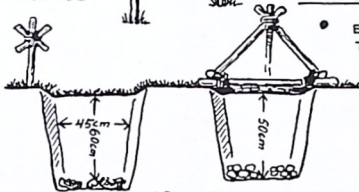
DETTE ER DET ABSOLUT MINSTE MÅL PÅ AFFALDSHUL OG FEDTFÆLDE, HVIS I VIL BEVARE HYGIEJEN I LEJREN
