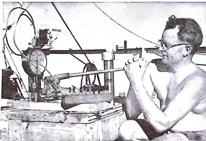
Professor Zo Bell med sit højtryksapparat, hvori han kan udsætte bakterierne fra de store dyb for et tryk, lige så stort som det, de kommer fra. Bakterierne holdes inde i en meget stærk stålcyllinder, som den, der ses midt i billedet
