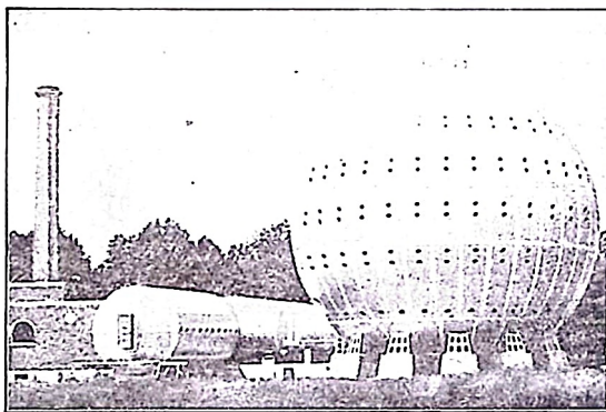
Dette er ikke en Ballon, men — et Hospital for Sukkersygepatienter ved Cleveland, Ohio. De syge lever i Staal-kuglen under et atmosfærisk Tryk, der er dobbelt saa stort, som det normale, og Behandlingen bestaar iøvrigt i, at der i Kuglen udvikles lidt i større Mængde. Der er 5 Etager i det mærkelige Hospital, som er 21 m i Diameter.
