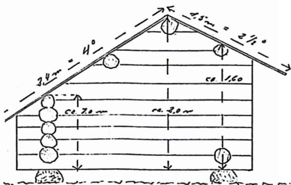
BJÆLKEVARK I SÅVLE. 1:25
