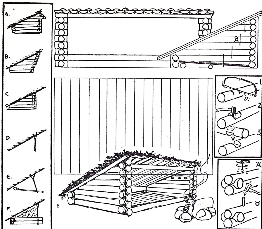
A: Meget solid — næsten som en hytte. B: Høje vægge, man kan stå oprejst i åbningen. C: Her er der sparet på tømmeret. D: Så enkel som mulig, blot et tag på to kløftede grene. E: Ligesom D, men med en stamme bagest og gulv. F: Ramme af tømmer og vægge af granbark.
