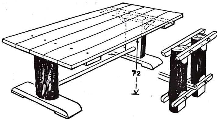
ALTMULIGMANDEN viser her et udmærket bord til jeres lokale. Bemærk at benene også kan laves som vist til højre.
