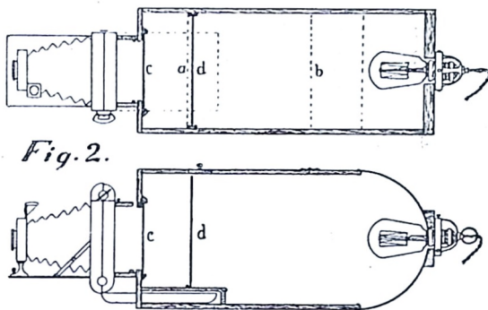
Fig. 2. Her ses et Snit af Kassen set henholdsvis fra oven og fra Siden. De punkterede Linjer a og b betegner Aabningen ind til Kassens Indre; c og d er Matskiverne.
