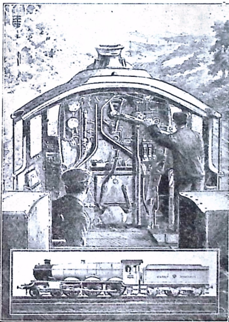
Paa Fyrpladsen paa »Den flyvende Skotte« i fuld Fart. Forneden ser man et Billede af Lokomotivet selv
