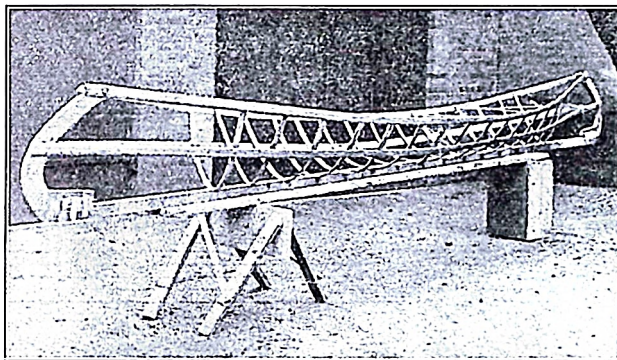
Skelet til en 4 m Kano
