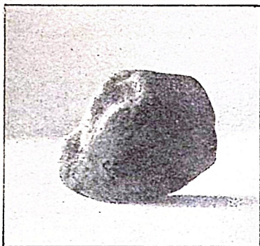
Metcorsten fra Pultuskfaldet d. 30 Jan. 1868. Tilhører Torvald Köhl, „Carina“, Odder. Den består af kulsur Kalk, Magnesia og Jern, vejer 42 Gram og har en Vægtfylde af 3,6.
