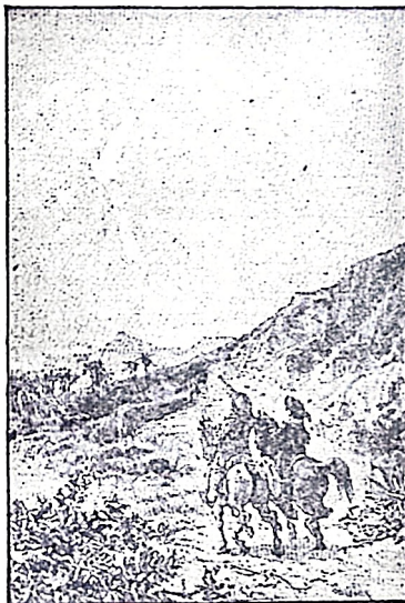
En Ildkugles Eksplosion i Brasilien.
