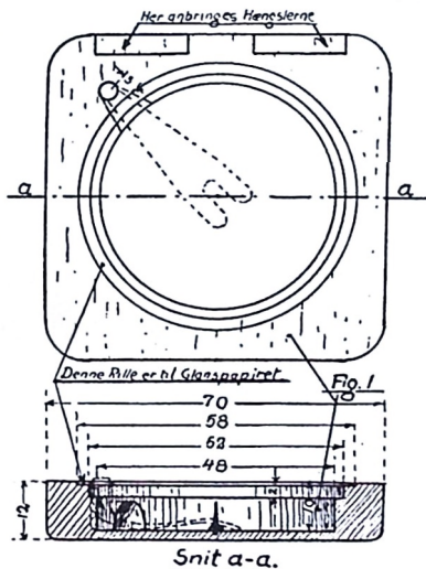
Arbejdstegning for Kompaskassen. 2/3 naturlig Størrelse. De angivne Maal er i mm.
