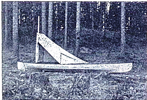
Langturskanoen „Y“, 4,20 0,70, Sejl: 3,7 m 2
