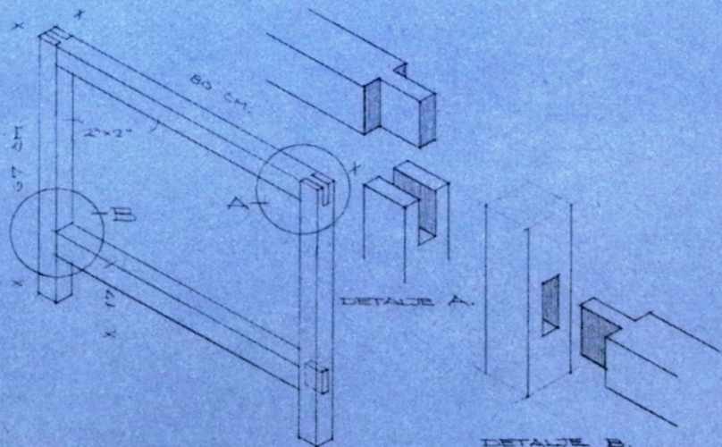
BORDEN MED DETALJER.
