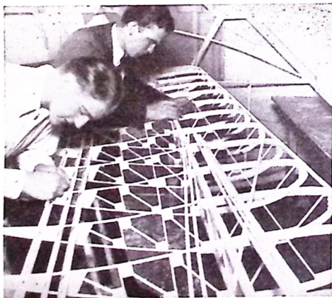
Med Flid og Energi bygger de fleste Klubber selv deres Svæveplaner.
