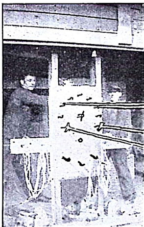
Maskinhuset. Man ser foroven 9 Kroge, af hvilke 4 er i Brug, forneden 3 til svævere Tovværk. De to Mænd drejer Haansvinget, der driver Krogene rundt.
