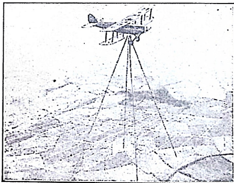
Et fotografisk Diagram, der viser, hvordan Fladerne bliver fotograferet saadan, at de gaar ind over hinanden, for at de bagefter kan sammenholdes.
