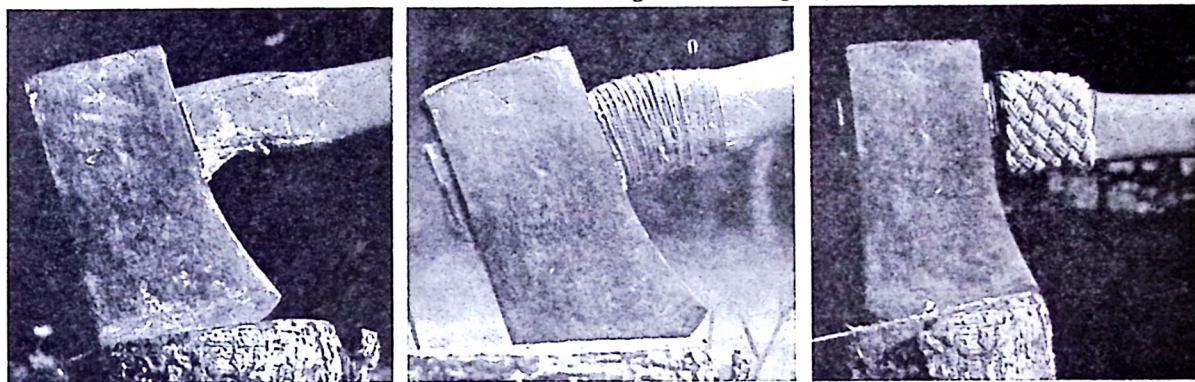
Fig. 5. Øksens svageste punkt kan beskyttes med et tyrkerknob. I dette tilfælde et tislået med ni bugter. Fremskredet slid og begyndende brud er her repareret med bændsling først.
