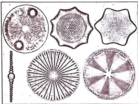
Mikroskopiske Billeder af smaa Alger, der lever oppe i de høje Luftlag, hvorfra de nu og da kommer ned som en Støvregn.
